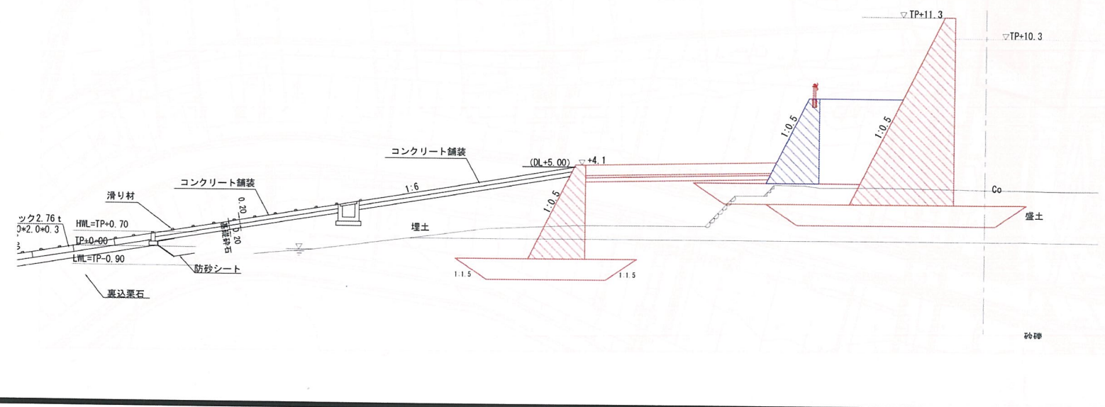
標準断面図
